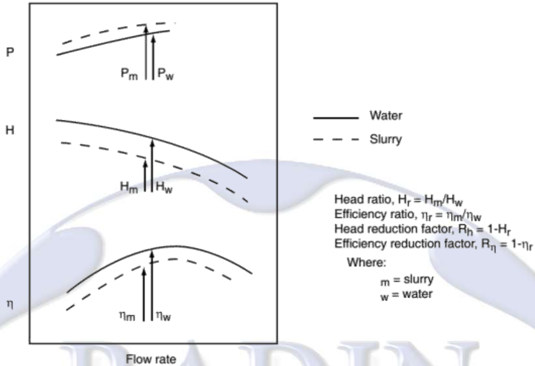
شکل ۴-۱: نمایش تاثیر اسلاری بر بازده و هد پمپ
