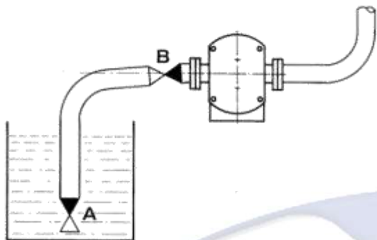
شکل ۲-۶: نمایش نحوه درست و نادرست مکش پمپ از مخزن
