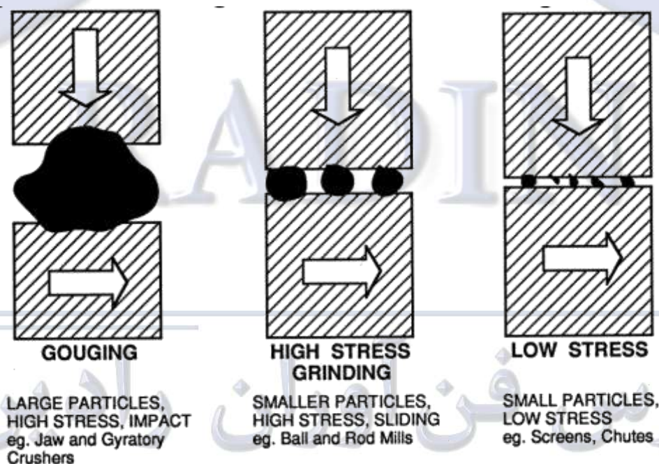
شکل ۳-۱: نمایش سه نوع از سایش Abrasion
